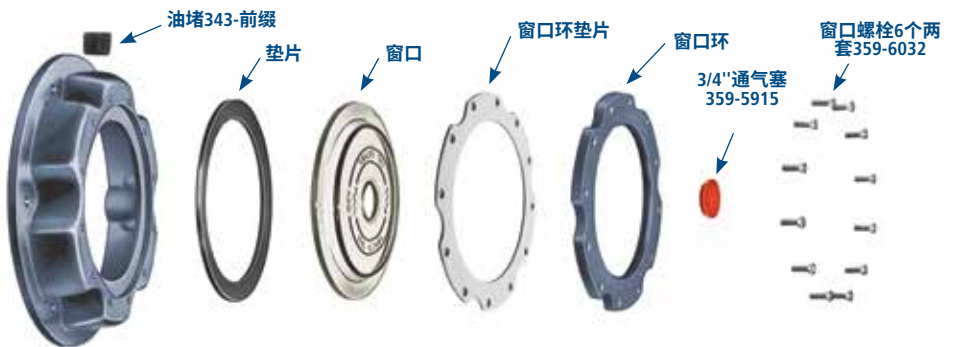
典型的4-3/8"窗口组件
