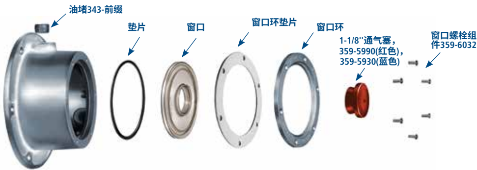
典型的2-3/4"和3-1/2"窗口组件
