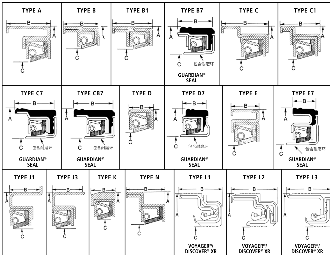
GUARDIAN®/GUARDIAN® HP 按零件号排序轮毂油封尺寸表
